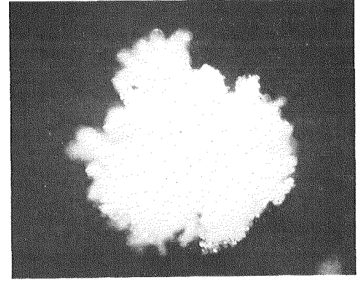
139 R4b Lump graupel \times 15
